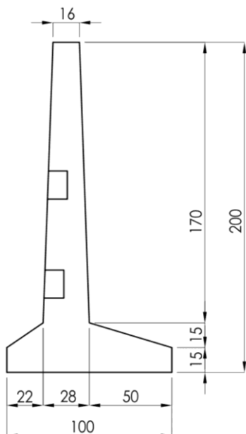
DETALLE VISTA
