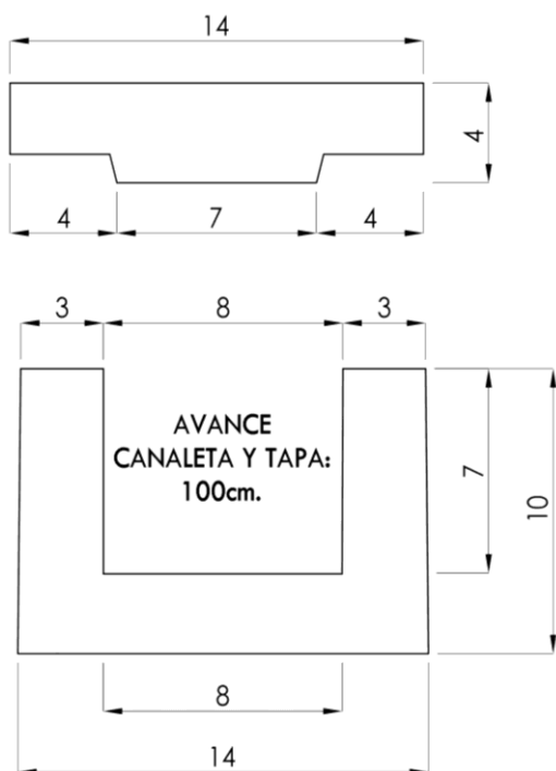
DETALLE VISTA
