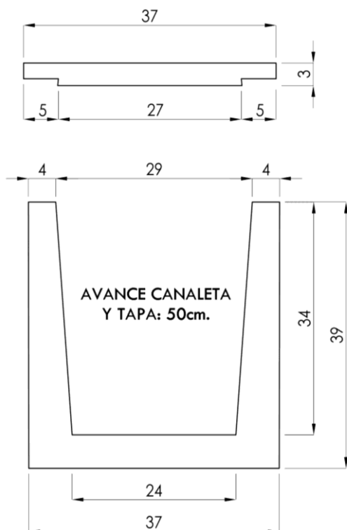
DETALLE VISTA
