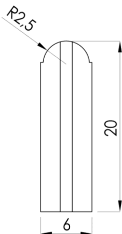
DETALLE VISTA
